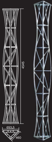
イカトラス
