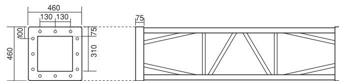
■ 主軸径 φ48.6mm / アルミニウム合金 ■ ボルト穴径 φ17.5mm × 12カ所
